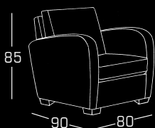
con piede quadrato (seduta più bassa di cm 3)
